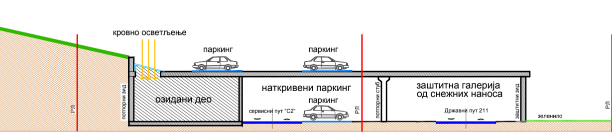
ПРЕСЕК А-А - КРОЗ ЗОНУ ГРАЂЕЊА У ОКВИРУ ГПО5
